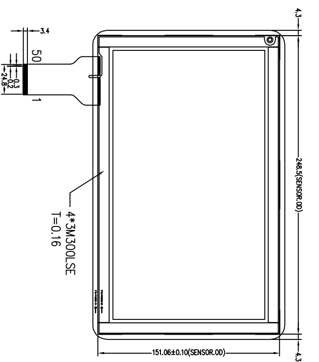
背面视图
