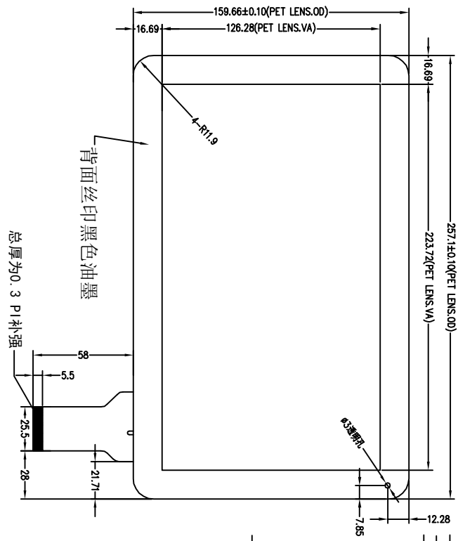
正面视图
